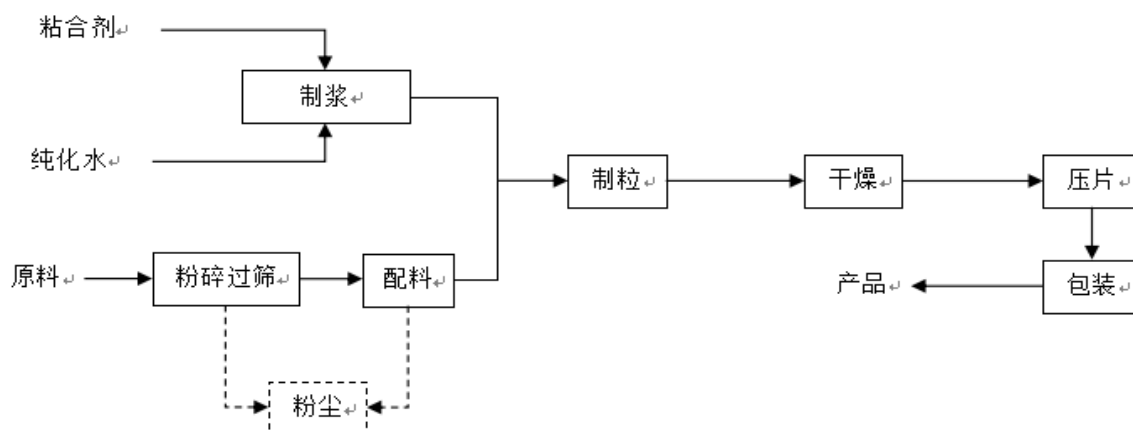
图 2-3 片剂颗粒剂工艺流程及产排污环节图
