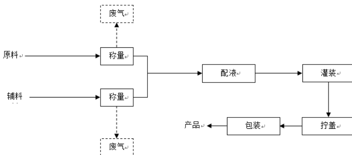
图 2-2 口服溶液剂工艺流程及产排污环节图
