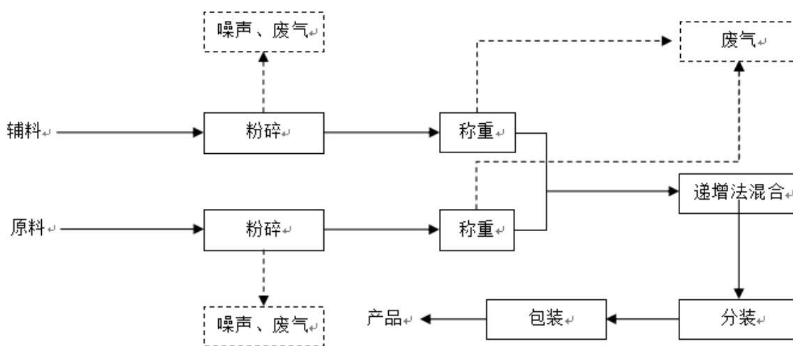
图 2-1 粉散剂工艺流程及产排污环节图
